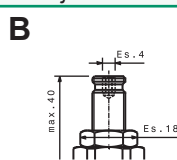
Vite esterna esagono incassato Leakproof hex socket screw
